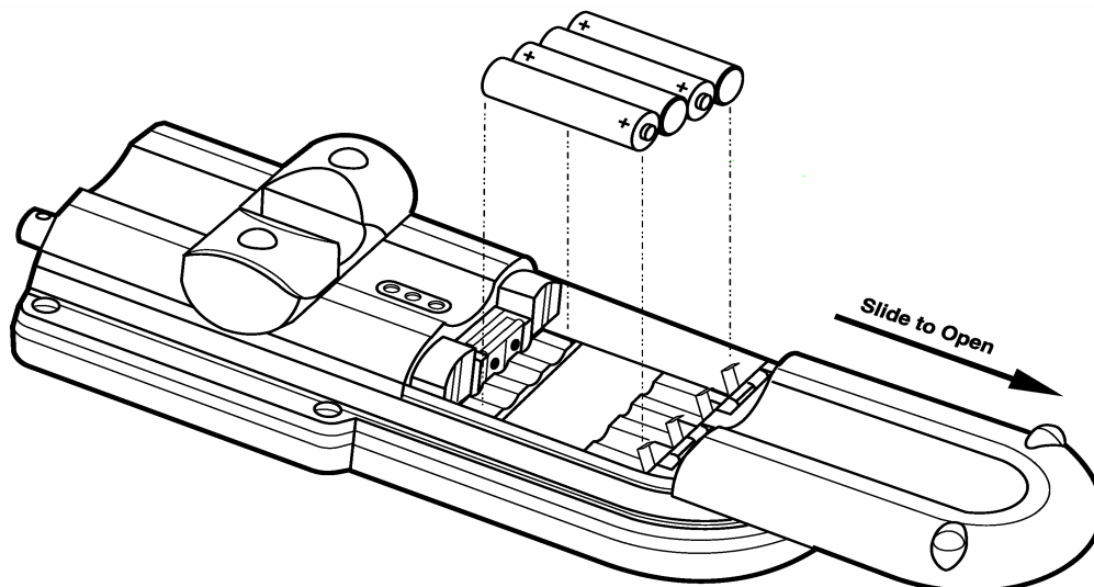
图 4 仪器电池安装
